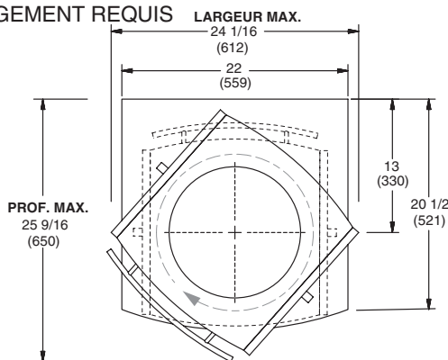
FIGURE 1. 0 VUE SUPÉRIEURE | DÉGAGEMENT REQUIS
