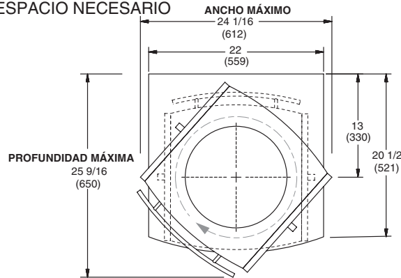
FIGURA 1. 0 VISTA SUPERIOR | ESPACIO NECESARIO
